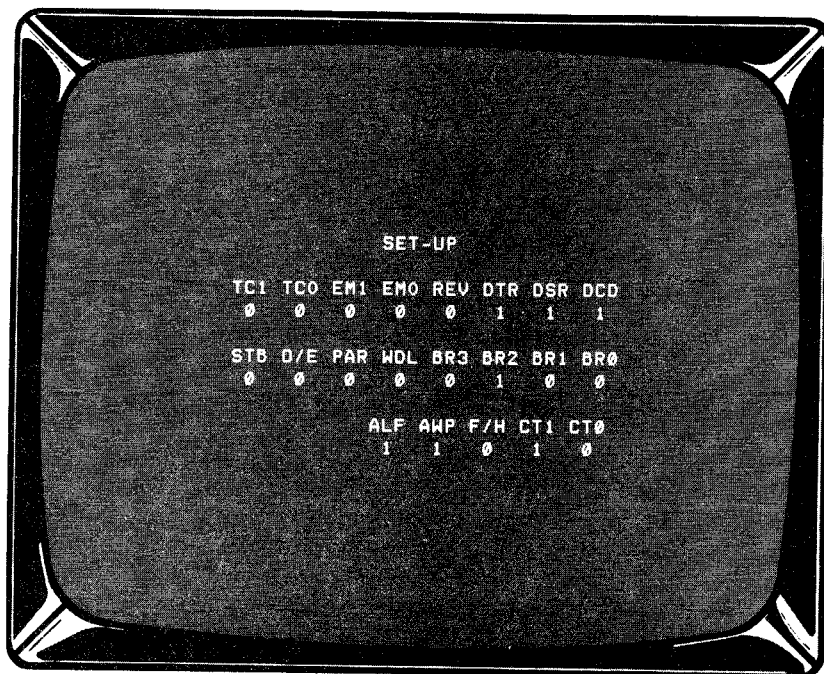
Figure 11. DT-1 I/O Parameter Menu
