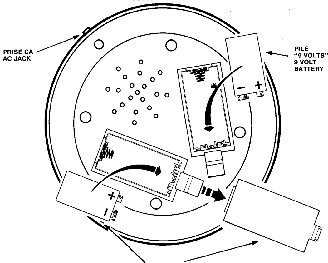
VUE DU DESSOUS DE L'UNITÉ BOTTOM VIEW OF UNIT
