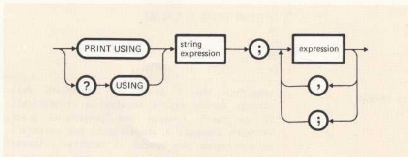
Figura 7-7 Istruzione PRINT USING
