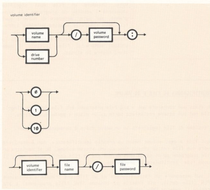
Figura 2-7 Identificatore di File e di Volume
