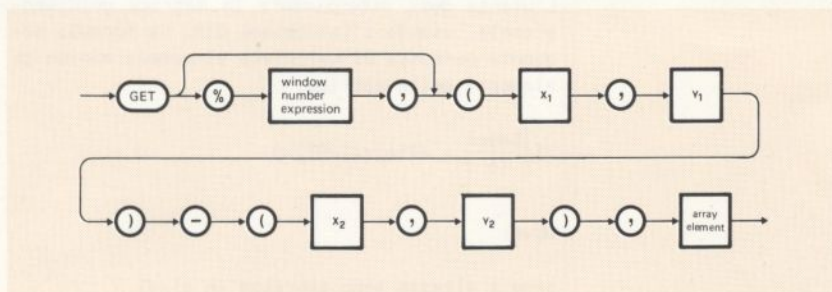
Figura 14-29 Istruzione GET - Grafica
