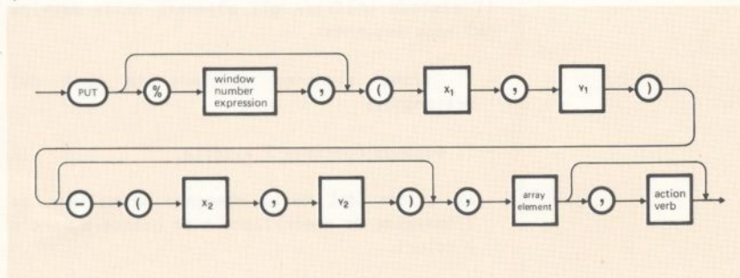
Figura 14-30 Istruzione PUT - Grafica
