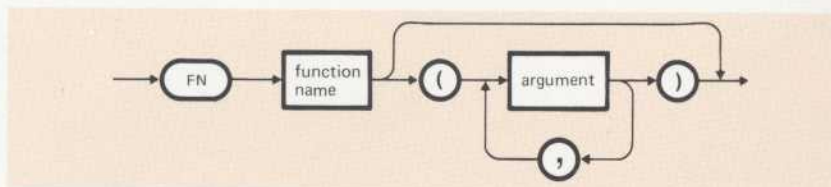
Figura 9-2 Richiamo della Funzione
