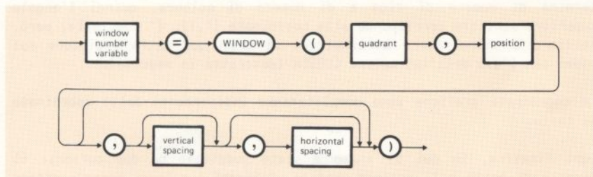
Figura 14-2 Istruzione WINDOW - Per aprire una finestra
