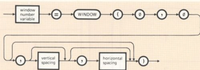
Figura 14-4 Istruzione WINDOW - Per variare lo spazio tra linee e caratteri
