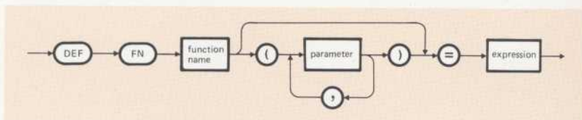
Figura 9-1 Istruzione DEF FN
