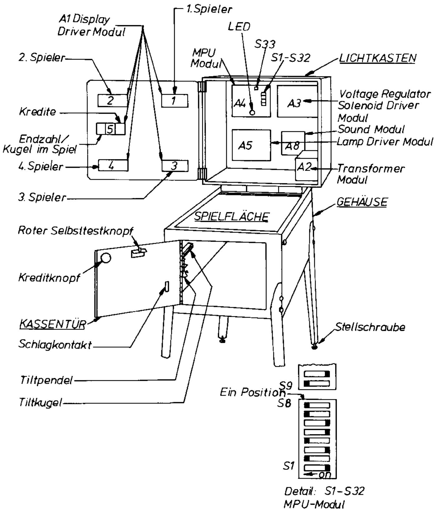
Abb. 2 Modullageplan
